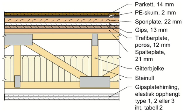
Fig. 4 Etasjeskiller med golvtipe 3
