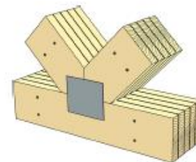
Fig. 1 Sammensatt takstolløsning med spikerplateforbindelser. Spikerplater mellom hvert staver og gurt.
