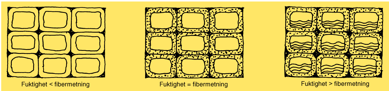
Figur 15.18 Skjematisk fremstilling av vedceller ved forskjellig fuktighet.
