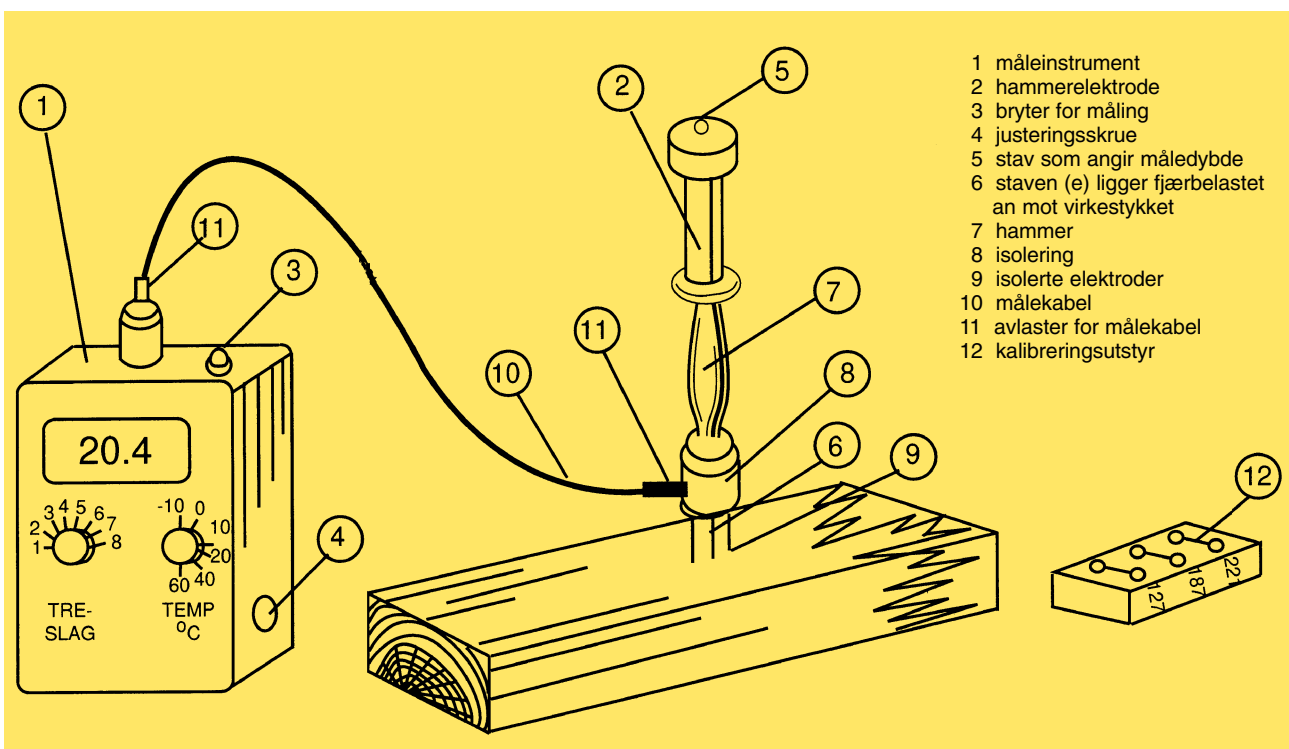
Figur 15.19 Elektrisk fuktighetsmåler av motstandstypen.
