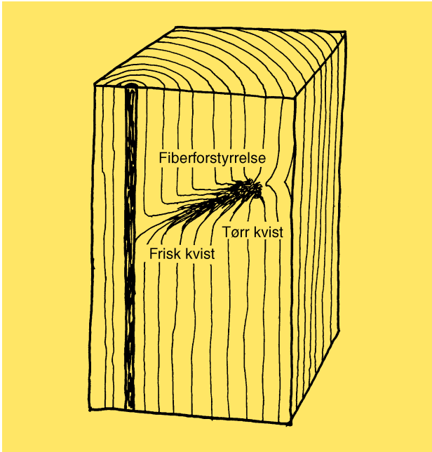
Figur 15.11 Kvistens innvirkning på vedstrukturen. Vi ser at kvistveden går omtrent på tvers av lengderetningen.
